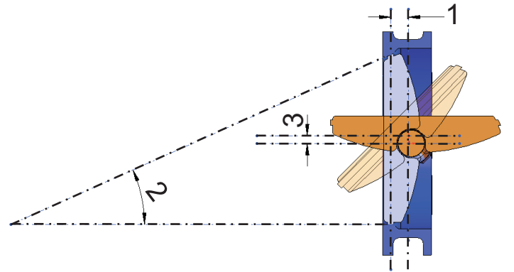
Üçlü Eksantrik Dizayn
