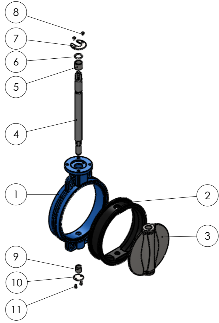
DN 250-300
